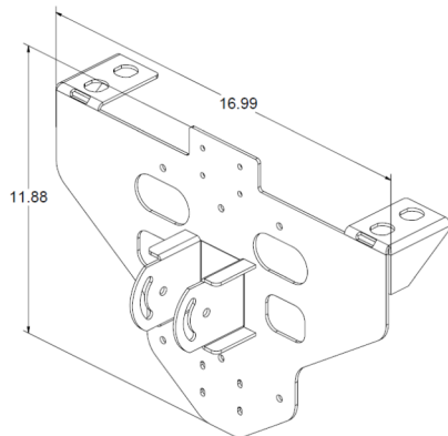
PTS5G-BK5111 & PTS5G-BK5114 1.8 lbs
